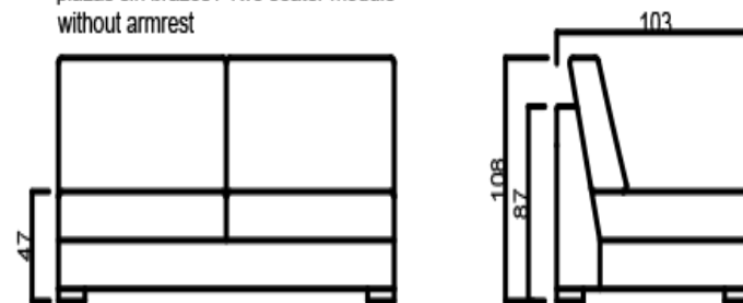
Módulo 2 lugares s/ brazo / Módulo de 2 plazas sin brazos / Two seater module without armrest
