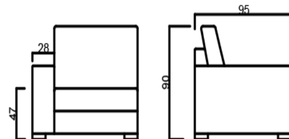
Módulo 1 lugar c/ 1 braço / Módulo de 1 plaza con 1 brazo / One-seater module with one armrest
