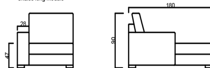
Módulo chaise long / Módulo chaise longue/ Chaise long module
