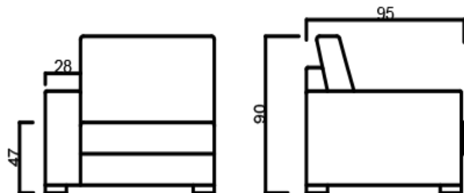
Módulo 1 lugar c/ 1 brazo / Módulo de 1 plaza con 1 brazo/ One-seater module with one armrest
