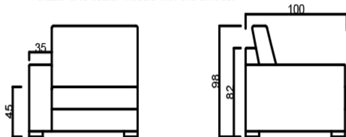
Módulo 1 lugar c/ 1 braço / Módulo de 1 plaza con 1 brazo/ One-seater module with one armrest
