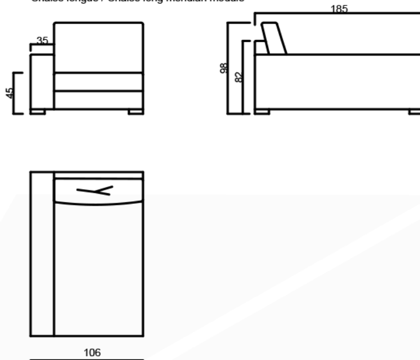
Módulo chaise long meridian / Módulo meridiano Chaise longue / Chaise long meridian module
